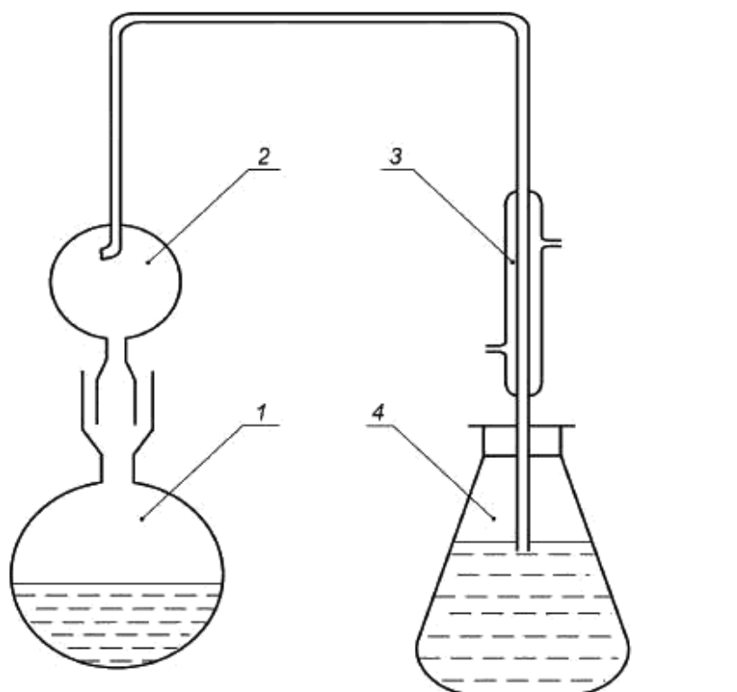
1 - круглодонная колба; 2 - каплеуловитель; 3 - холодильник; 4 - приемная колба
